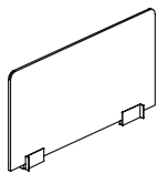
PRZEGRODA TAPICEROWANA WYSOKOŚĆ 800MM, GR: 42MM KOLORY: PRÓBNIK
